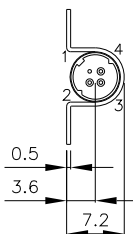
Horizontal Flange
