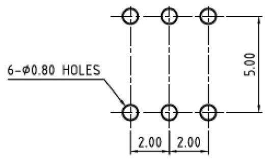
P.C.B DIMENSION
